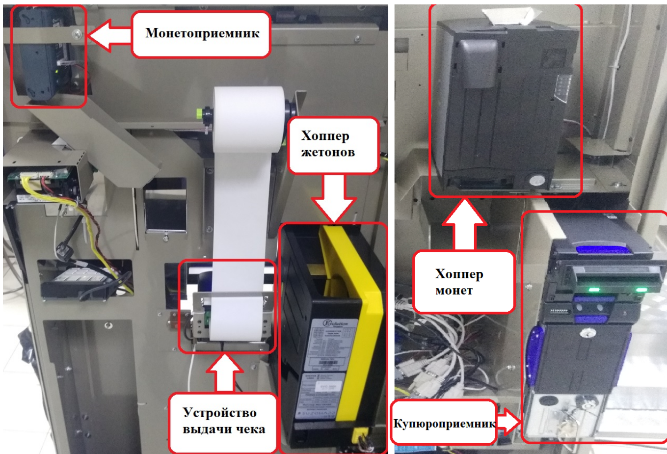
Внутреннее устройство терминала
